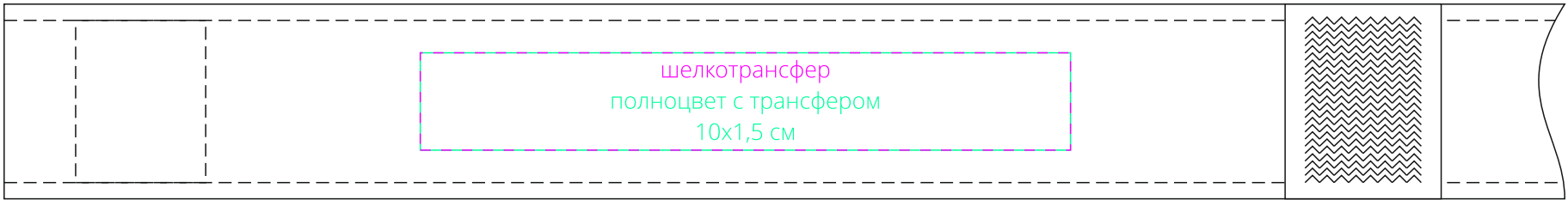
хлястик (зонт в закрытом виде) M1:1
