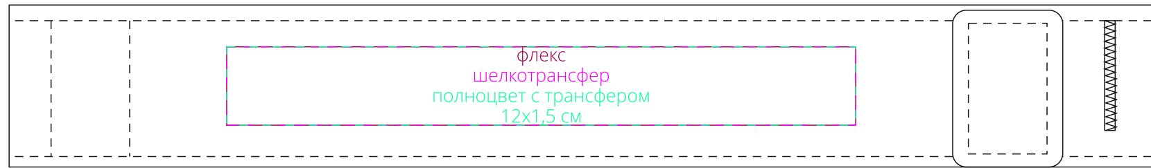
хлястик (зонт в закрытом виде) M1:1
